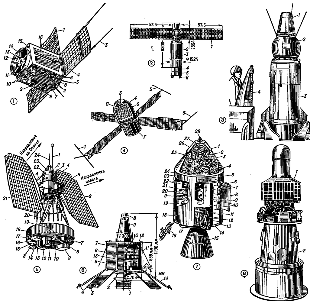
Рис. 1. Спутник ITOS-1. 1 — панель с солнечными элементами; 2 — телевизионные камеры системы АРТ; 3 — антенны (137,5 Мгц); 4 — механизм, обеспечивающий раскрытие панели с солнечными элементами; 5 — антенна командного приемника (148,5 Мгц) и радиомаяка; 6 — датчик направления на Землю; 7 — турбинетная антенна; 8 — датчик направления на Солнце; 9 — телевизионные камеры системы AVCS; 10 — радиометры SA; 11 — радиометр для измерения альbedo Земли; 12 — датчик горизонта; 13 — маховик; 14 — плоскость разделения спутника и последней ступени ракеты-носителя; 15 — прибор SPM для регистрации протонной составляющей солнечной излучения; 16 — жалюзи системы терморегулирования. Рис. 2. Спутник SERT-II с ракетой «Аджона Дн». 1 — панель с солнечными элементами; 2 — ракета «Аджона Дн»; 3 — центр масс объекта, обращающегося по орбите; 4 — вспомогательный отсек спутника SERT-II; 5 — основной отсек спутника; 6 — ионный двигатель (2). Рис. 3. Спутник «Оузма». 1 — приборный контейнер; 2 — четвертая ступень ракеты-носителя (РДТТ с шаровидным корпусом); 3 — третья ступень ракеты-носителя; 4 — часть головного обтекателя. Рис. 4. Спутник «Эксplorер XII». 1 — телеметрическая антенна; 2 — звездный датчик; 3 — устройство для включения звездного датчика; 4 — солнечный датчик; 5 — командная антенна; 6 — блок научной аппаратуры; 7 — блок служебной аппаратуры. Рис. 5. Спутник «Нимбуд IV». 1 — выдвигная стержень гравитационной системы ориентации и стабилизации; 2 — заправочный штуцер пневматической системы; 3 — реактивное сопло для ориентации по тангажу; 4 — солнечный датчик; 5 — датчик горизонта; 6 — панель со штепсельными разъемами; 7 — радиометры SCR; 8 — антенна диапазона S; 9 — спектрометр IRIS; 10 — антенна системы IRLS; 11 — радиометр THIR; 12 — спектрометр SIRS; 13 — спектрометр BUVS; 14 — телевизионная камера IDC; 15 — детектор MUSE; 16 — датчик ультрафиолетового излучения, используемый в радиометрах SCR; 17 — спектрометр FWS; 18 — контейнер с научными приборами и телевизионными камерами; 19 — антенны (4) радиомаяка; 20 — элемент конструкции; 21 — панель с солнечными элементами; 22 — реактивное сопло для ориентации по рысканию; 23 — реактивное сопло для ориентации по крену; 24 — антенна командной системы. Рис. 6. Спутник «Пвож». 1 — устройство для образования стержня гравитационной системы ориентации; 2 — трехосный датчик колебаний; 3 — солнечные датчики; 4 — отражатели лазерного излучения; 5 — электромотор, обеспечивающий развертывание стержня гравитационной системы ориентации и стабилизации; 6 — магнитометр; 7 — аккумуляторная батарея; 8 — датчик, используемый для определения альbedo; 9 — коническая спиральная антенна; 10 — датчик пороговой перегрузки (30 g); 11 — антенна командно-телеметрической системы; 12 — элемент амортизирующей подвески аппаратуры;
