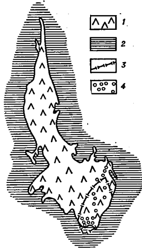
Рис. 1. Жемпирсайский ультраосновной хромитовый массив: 1 — ультраосновные породы, 2 — вмещающие породы, 3 — контур проекции магмоподводящего канала, 4 — месторождения хромитов в юго-восточной части массива.
