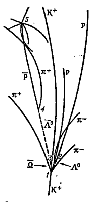
Схематическое изображение распада антамегагиперона \bar{\Omega} .
