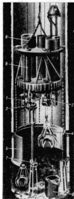
Рис. 1. Схема проходки ствола с использованием комплекса 2КС-1 м: 1 — радиальная рама; 2 — кабина машиниста; 3 — пневмотельфер; 4 — грейфер; 5 — передвижная опалубка; 6 — саморазгружающаяся балка; 7 — буровая установка БУК-1м; 8 — бетонораспределитель; 9 — двухэтажный подвесной полк.
