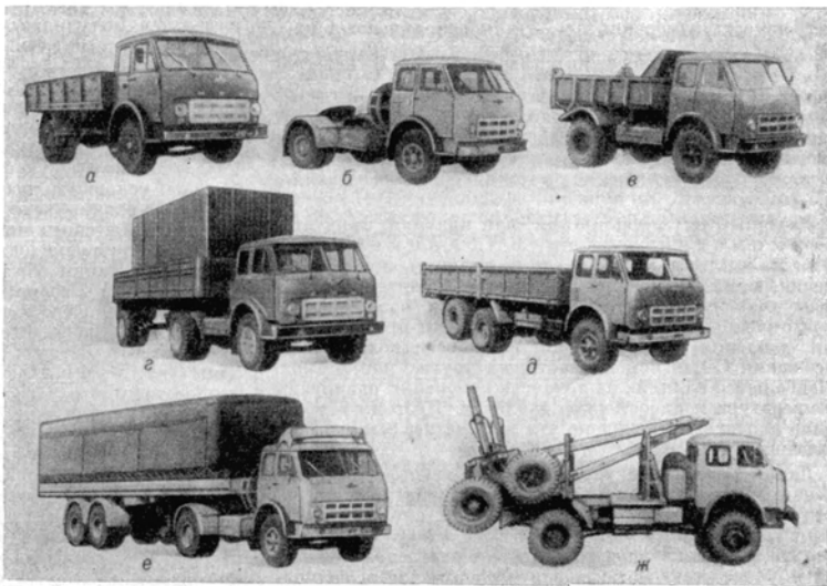
Рис. Автомобили семейства МАЗ-500: а — МАЗ-500А; б — МАЗ-504А; в — МАЗ-503А; г — МАЗ-504А-3245; д — МАЗ-516; е — МАЗ-504В-5205; ж — МАЗ-509.
