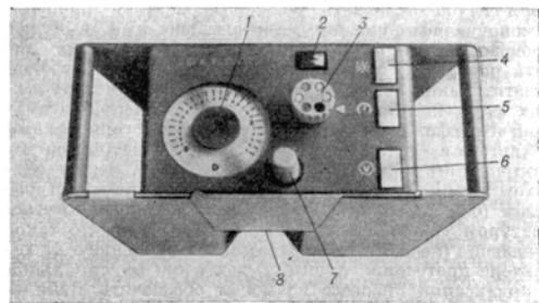
Рис. 4. Денситометр Д-1 фирмы «Гретаг»: 1— измерительная шкала; 2— индикатор нагрузки; 3— переключатель фильтров; 4 — кнопка включения светового пята; 5 — кнопка измерения; 6 — кнопка контроля нагрузки; 7 — ручка калибровки; 8 — измерительная площадка.
