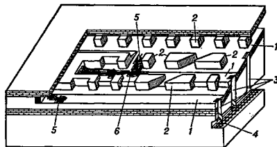
Рис. 4. Четвертый комплекс: 1 — камеры; 2 — опорные цепяки; 3 — рудоспуск; 4 — штырь; 5 — буровые каретки; 6 — погрузочная машина.
