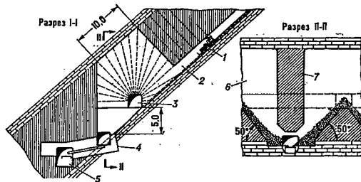
Рис. 3. Третий комплекс: 1 — буровая каретка; 2 — разрезной возстающий; 3 — буровой штырь; 4 — шпрт; 5 — откаточный штырь; 6 — камера; 7 — опорный ленточный цепик.
