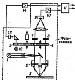
Рис. 3. Инфракрасный измеритель: 1— источник излучения; 2— оп-объектив; 3— печатная форма; 4— вращающийся обтюратор; 5— вспомогательный обтюратор; 6— природный двигатель; 7, 8— фильтры; 9— приемник излучения; 10— предварительный усилитель; 11— выходной преобразователь; 12— вспомогательный источник излучения; 13— фотодиод; 14— усилитель.
