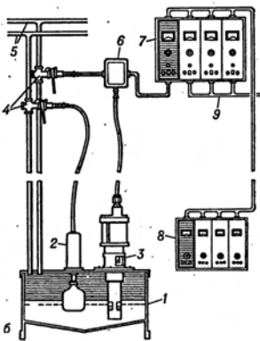
Рис. 2. Прибор «Вискомекс-384». Общий вид (а) и (б) схема: 1 — бачок для краски; 2 — регулятор уровня краски в бачке; 3 — измеритель вязкости краски; 4 — пневматические клапаны; 5 — трубопроводы для подачи краски и растворителя; 6 — узел пневматического клапана; 7 — панель управления; 8 — шкаф управления; 9 — кабель (к др. печатным секциям).
