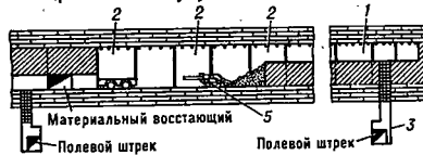
Рис. 2. Второй комплекс: 1 — камеры; 2 — опорные целики; 3 — рудоспуски; 4 — буровая каретка; 5 — погрузочная машина.
