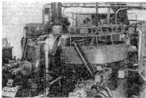
Рис. 2. Внешний вид установки ВЭПП-2.
