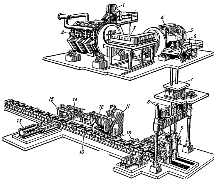
Автоматизированная линия непрерывного получения вафербаров из бескислородной меди: 1—загрузочная машина; 2—электродуговая индукционная печь ИЛМ-16м01; 3—обогреваемый переливной желоб; 4—индукционный мисер ИЛОМ-2,5; 5—разливочная корoba; 6—блок кристаллизаторов с камерой вторичного охлаждения; 7—линейная клетка; 8—летучая плита; 9—наплавочный слиток; 10—магистральный ролик с приводными роликами; 11—пила для разрезки слитков на конечный размер; 12—участок контроля; 13—гидрокаталител; 14—штабелерщик с клеймителями; 15—готовые слитки.
